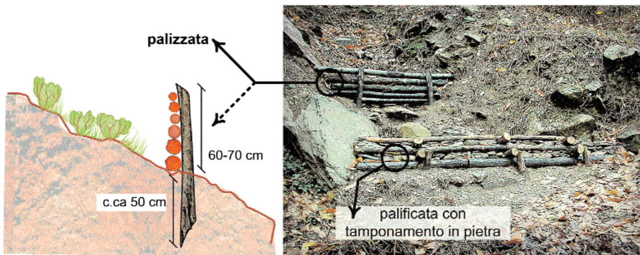
Fig. 31 - Mutamenti del paesaggio terrazzato del Monte Pisano. Esempio di palizzata a confronto con la palificata. [Schema e foto: F. Casella]
