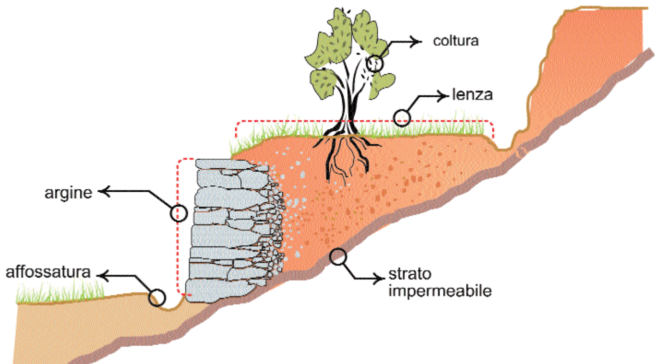
Fig. 21 - Terrazzamenti. Schema degli elementi costitutivi del terrazzamento: argine, lenza e affossature. [Schema: F. Casella]
