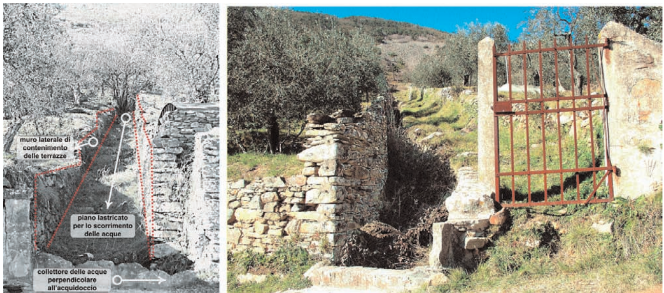
Fig. 20 - I canali di drenaggio. Schema e foto di acquidoccio. Da notare le dimensioni ristrette della sezione e la forte pendenza del piano di scorrimento. Entrambe queste caratteristiche rendono difficoltoso l'uso di mezzi meccanici per la gestione. [Foto: D. Rizzo]
