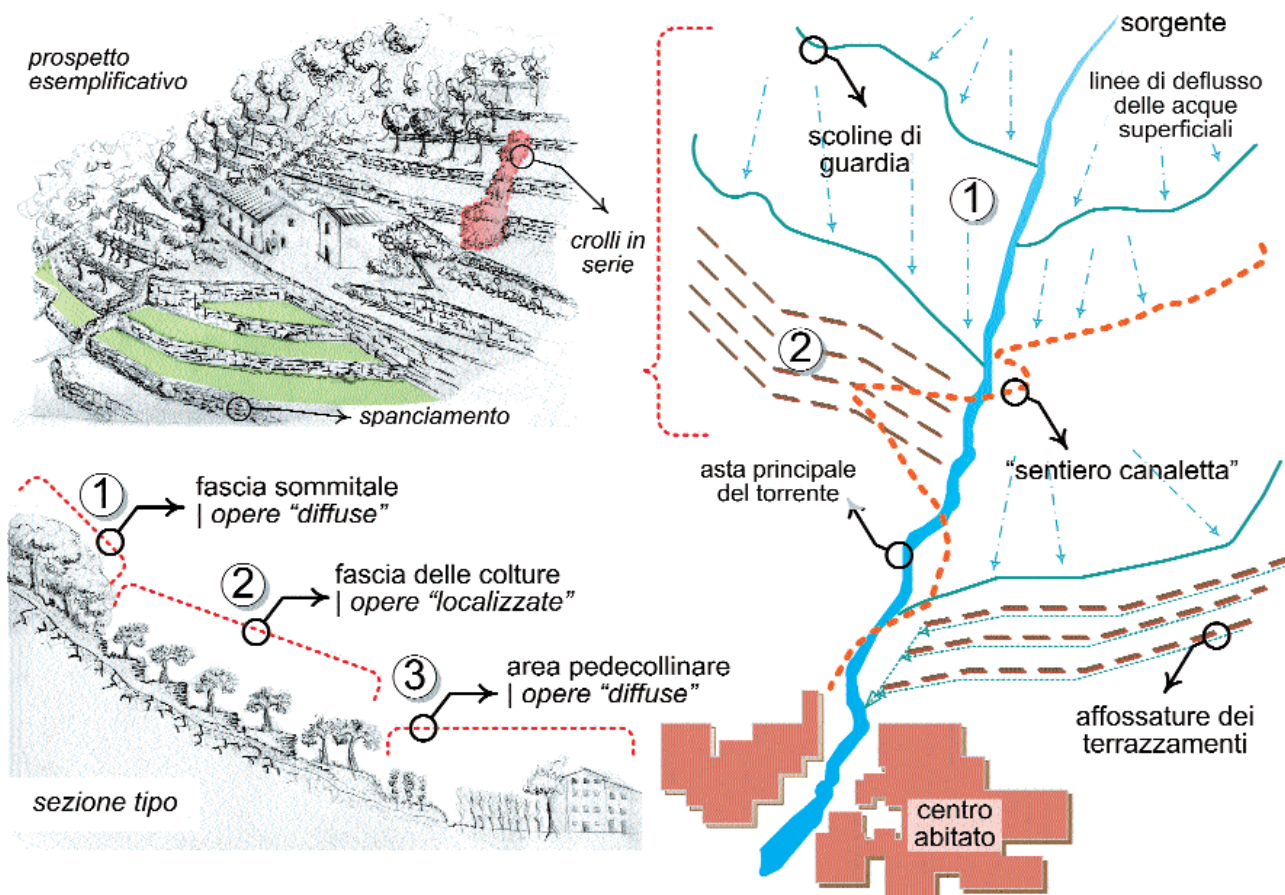
Fig. 17 - Sistema idraulico agrario e forestale del Monte Pisano. Descrizione schematica delle tre macro-aree principali. [Schema: F. Casella]
