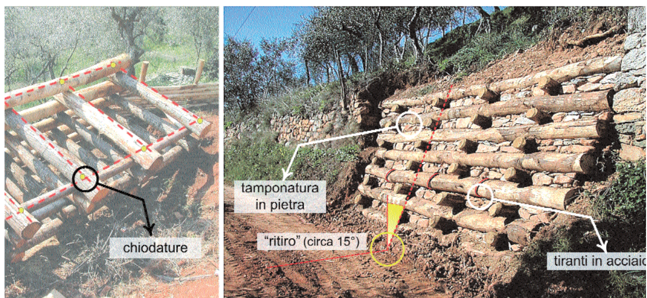
Fig. 32 - Mutamenti del paesaggio terrazzato del Monte Pisano. Dettagli strutturali della palificata doppia. [Schema: F. Casella e D. Rizzo]
