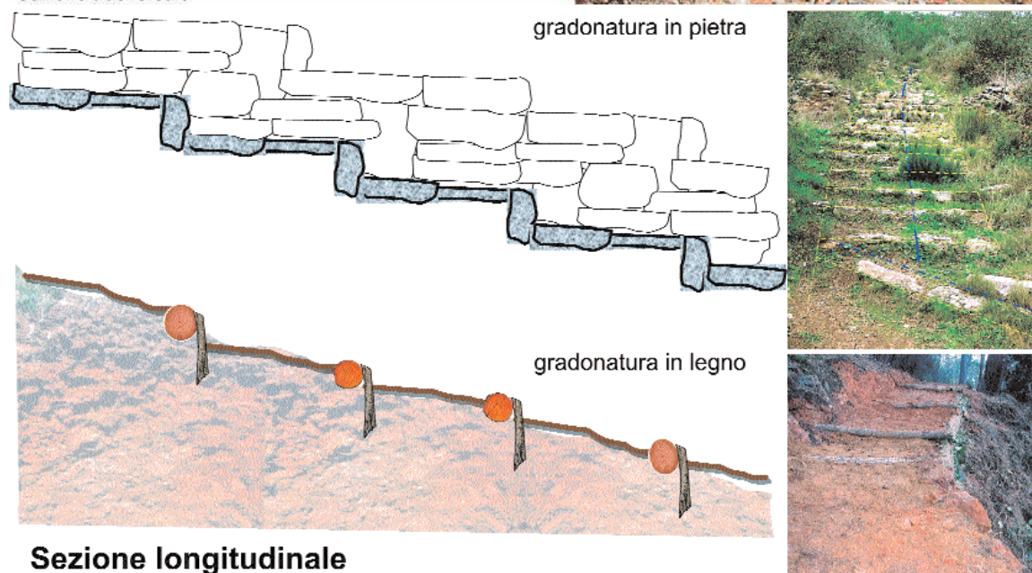
Fig. 19 - I canali di drenaggio. Le principali tipologie dei percorsi idraulici individuabili sul Monte Pisano. (a) Sezione longitudinale e trasversale di sentiero lastricato a impluvio centrale; (b) sezione longitudinale e trasversale di sentiero lastricato a impluvio laterale; (c) sezione longitudinale di sentiero con gradonatura in pietra e in legno. [Schemi e foto: F. Casella]
