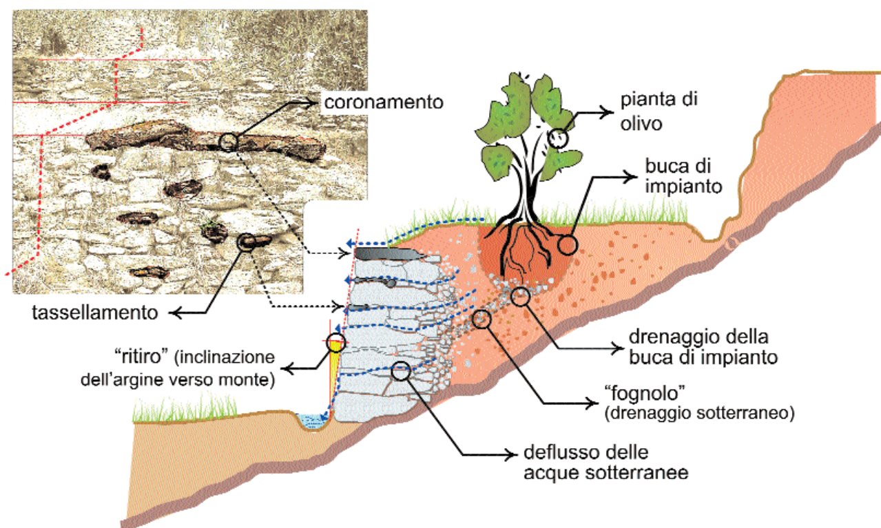
Fig. 22 - Terrazzamenti. Argine in muratura a secco, componenti della struttura e schema delle funzioni. [Schema: F. Casella; D. Rizzo]
